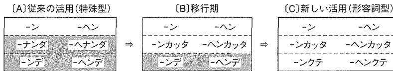
図8 否定辞活用体系の形容詞化
