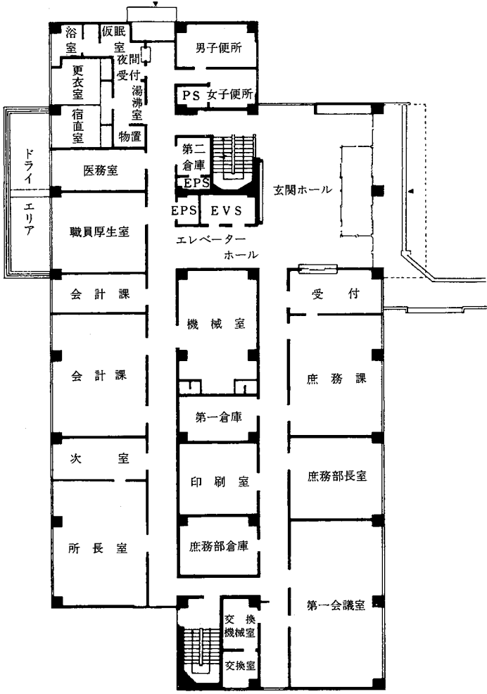
1階平面図
