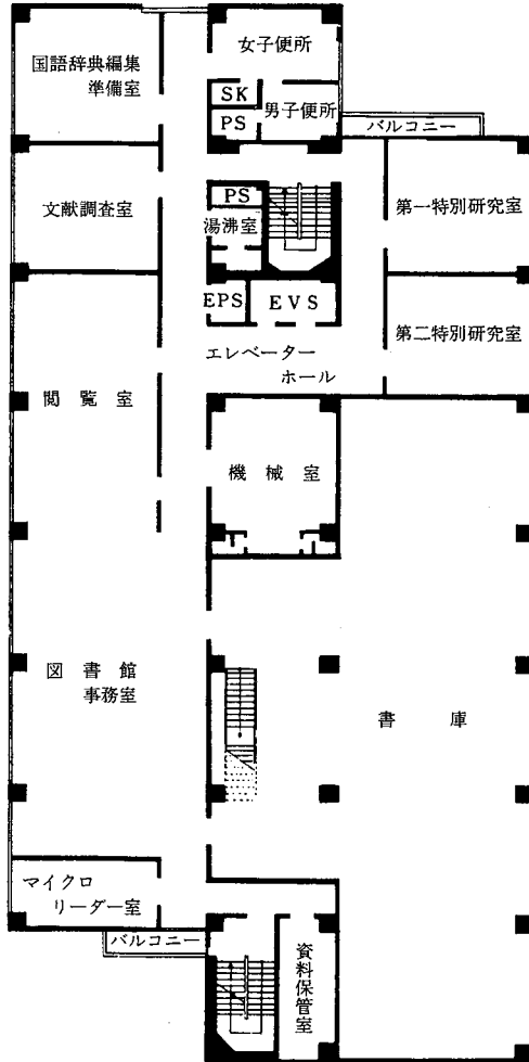
3階平面図
