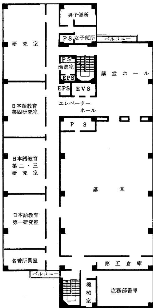
5 階平面図
