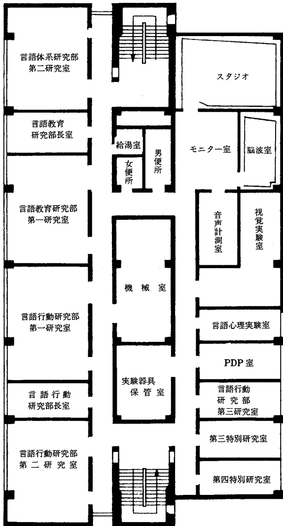
3 階平面図
