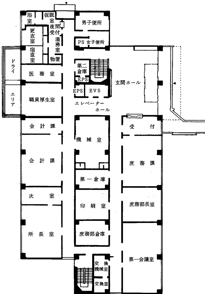
1階平面図
