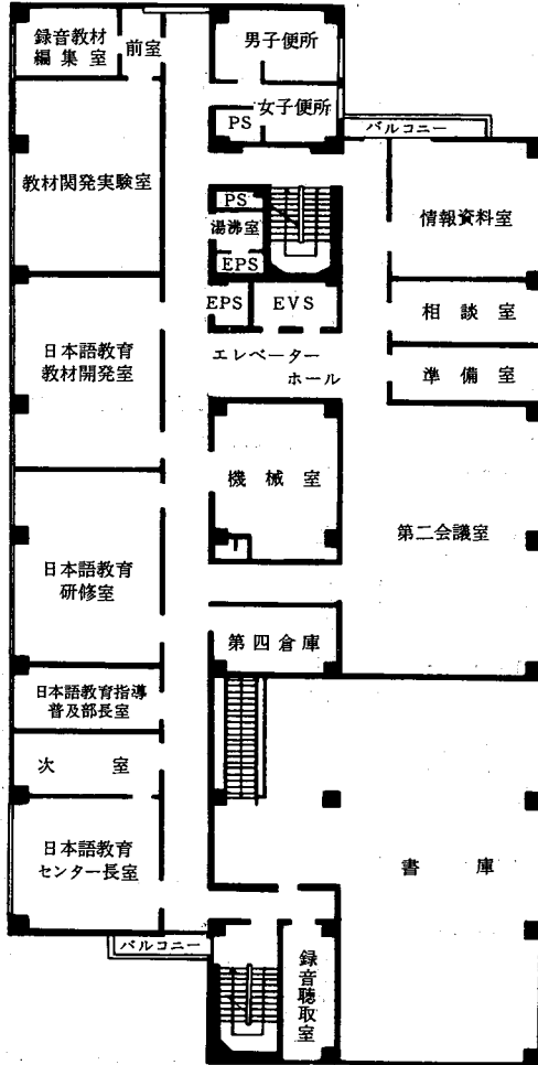
4階平面図
