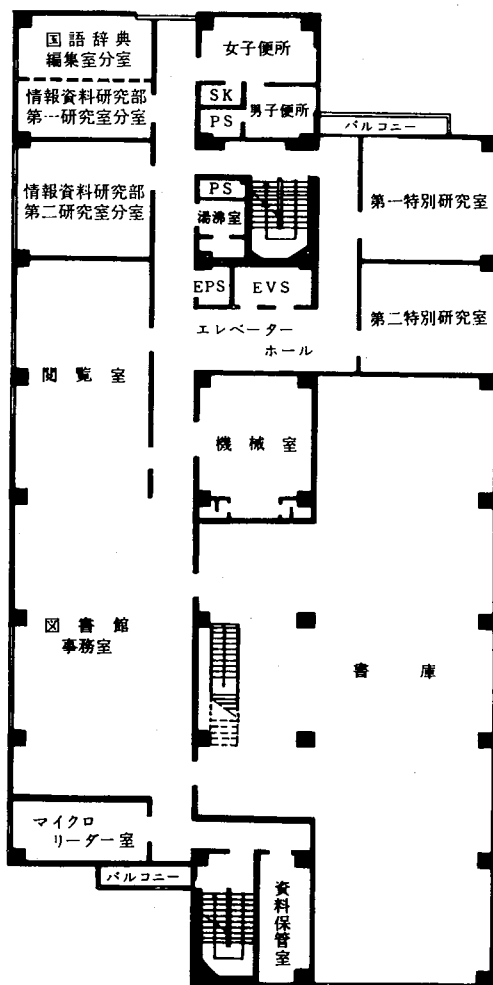
3階平面図
